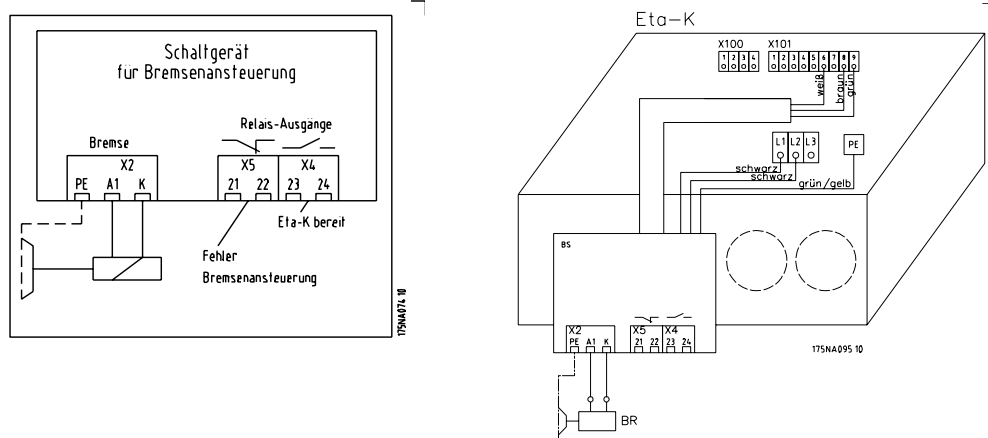
Abbildung 5.1: Elektrischer Anschluss der Bremsansteuerung an Eta-K
