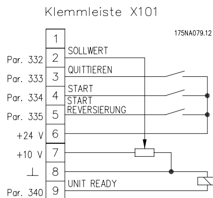
Abbildung 3.1: Der Wert eines externen Sollwertpotentiometers muss zwischen 1 kOhm und 5 kOhm betragen.
