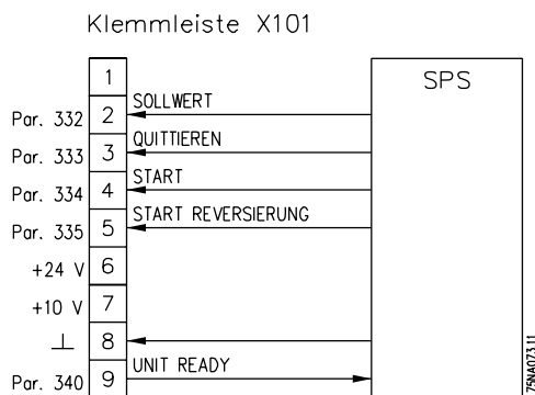
Abbildung 3.2: Steuersignale von SPS
