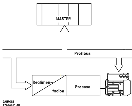
Lazo de control cerrado en el bus
