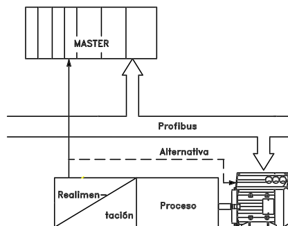
Cierre del lazo de control fuera del bus para una realimentación muy rápida
