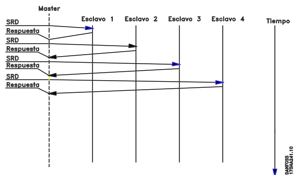
Transmisión cíclica rápida con PPO utilizando DP
