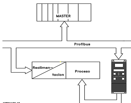
Transmisión cíclica rápida con PPO utilizando DP
